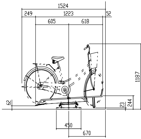
側面図 S = 1 / 20
